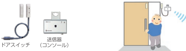
Dタイプセンサーセット(ドアスイッチ+送信器) HK-3DS
