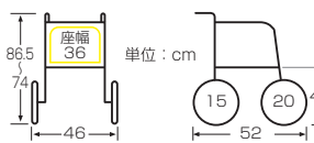
●折りたたみ時
