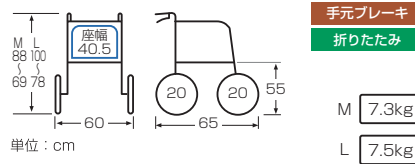
●折りたたみ時
